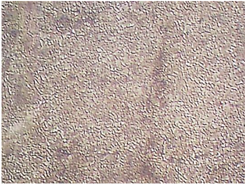
Рис. 5 – Структура стали 40 после улучшения, \times 200
